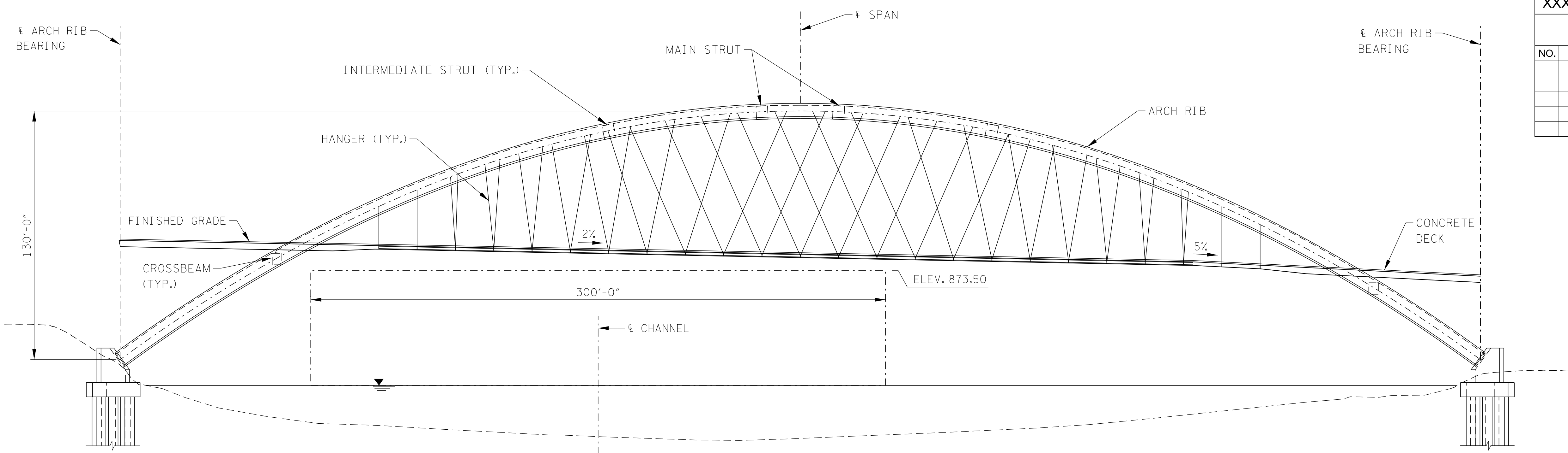
ELEVATION SCALE: 1' = 380'-0"
